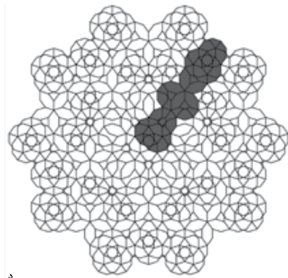
تصویر ۲۰- الف، تصویر عنصر سیلیکون در حالت شبه بلوری - ب، انطباق ۱۰ ضلعی‌های منتظم بر روی ساختار سیلیکون - ج، ترسیم ساختار سیلیکون متشکل از تلاقی ۱۰ ضلعی‌های منتظم - د، نمایش تلاقی ۱۰ ضلعی‌های منتظم با نظم شبه بلوری.
