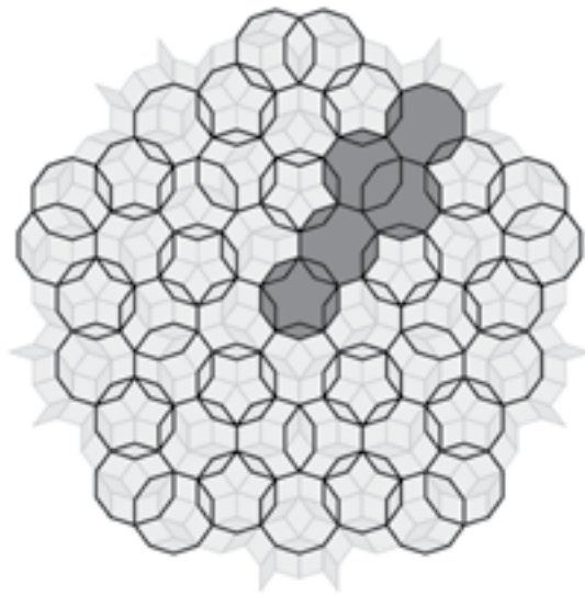
تصویر ۱۰- چیدمان ۱۰ ضلعی‌های متداخل در یکدیگر به صورت شبه تناوبی منطبق بر کاشیکاری پنزوز.
