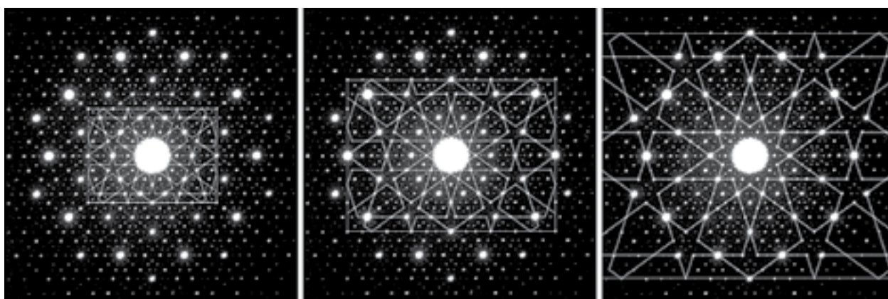
تصویر ۱۸- انطباق گره تند دو پنج در سه مقیاس مختلف بر تصویر پراش پراگ از آلیاژ AL_{70}Ni_{15}Co_{15} .
